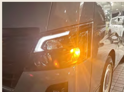
純正ヘッドランプ ウィンカー LED 化 IPF LED ウィンカー (501WB) + 抵抗 (WA19) ※取付工賃込み
