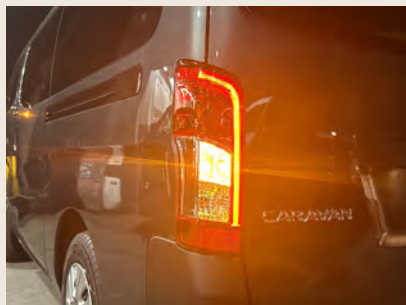
純正テール ウィンカー&バックランプ LED 化 IPF LED ウィンカー (501WB) + 抵抗 (WA19) + LED バック (703BL) ※取付工賃込み
